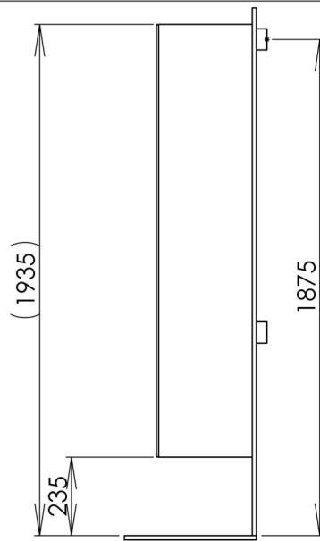
Högskåp/High cabinet/Korkeakaappi
