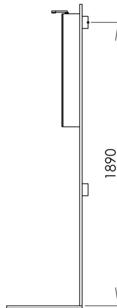
Spegelskåp/Mirror cabinet/Peilikaapit
