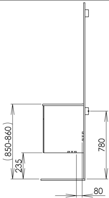
Underskåp/Vanity unit/Allaskaapit
