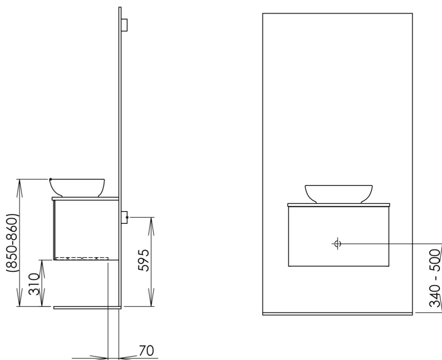
Underskåp/Vanity unit/Allaskaapit
